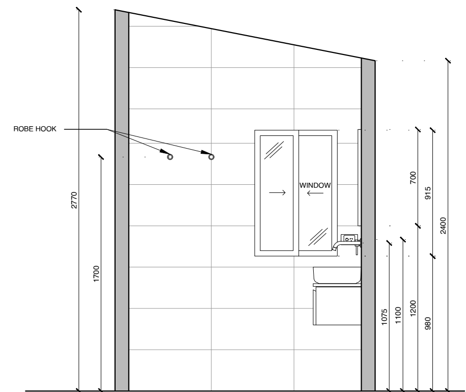
ELEVATION - 4
