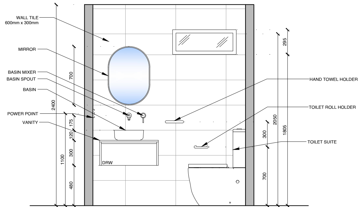
ELEVATION - 1
